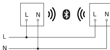
Schema elettrico Master-Master collegamento in rete
